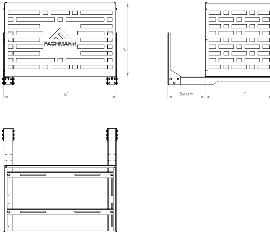
Рис. 1. Размеры корзины для кондиционера.
